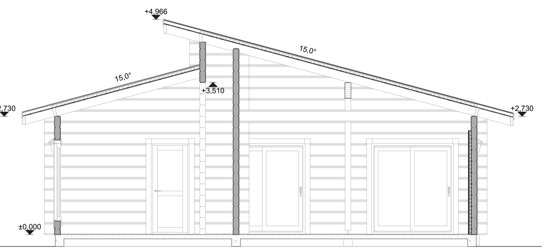
C SECTION C-C leikkaus
