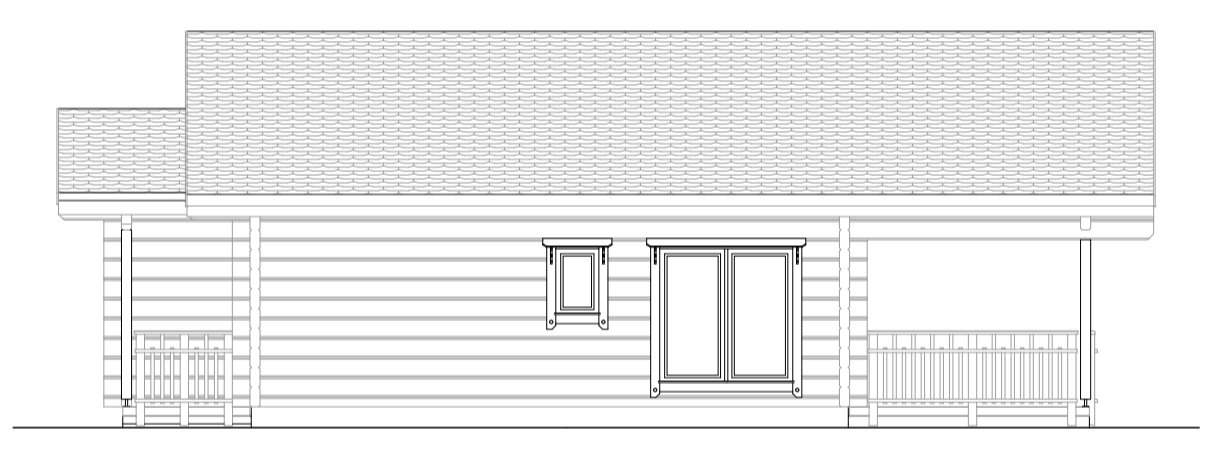
2 ELEVATION H-A juoksisivu
