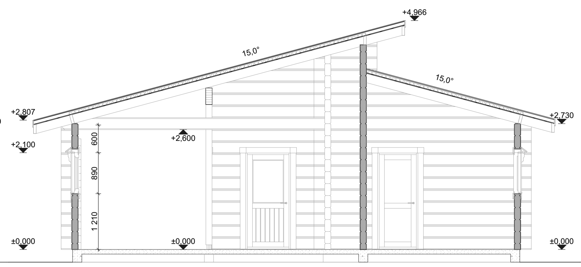
B SECTION B-B leikkaus
