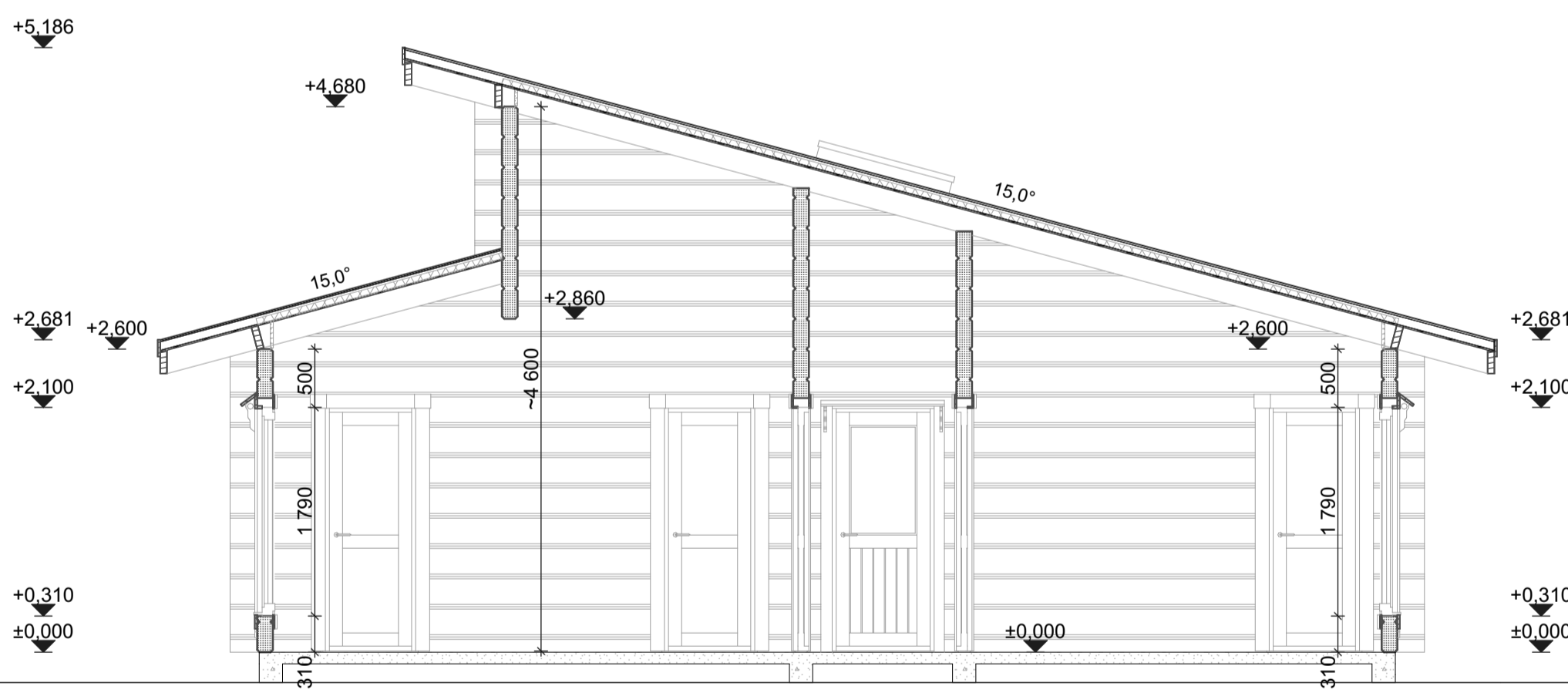
D SECTION D-D leikkaus
