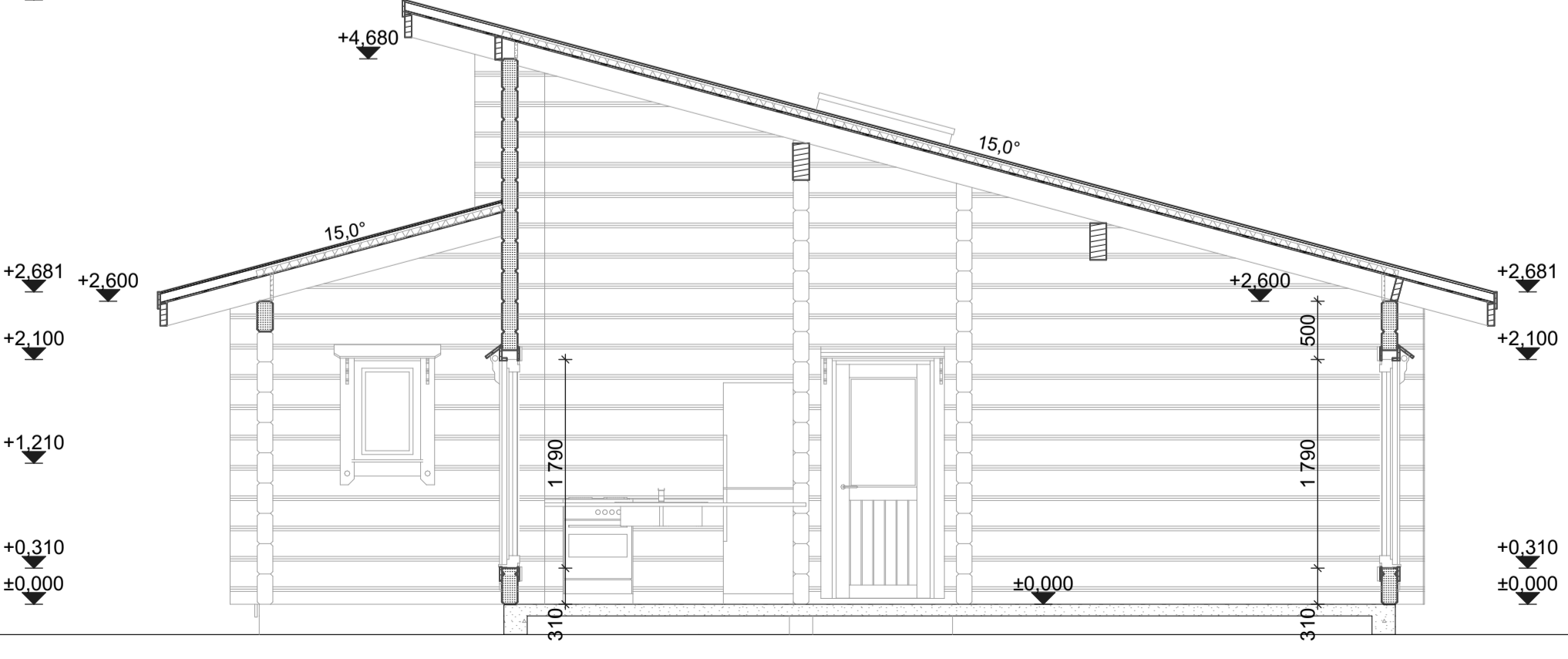
C SECTION C-C leikkaus
