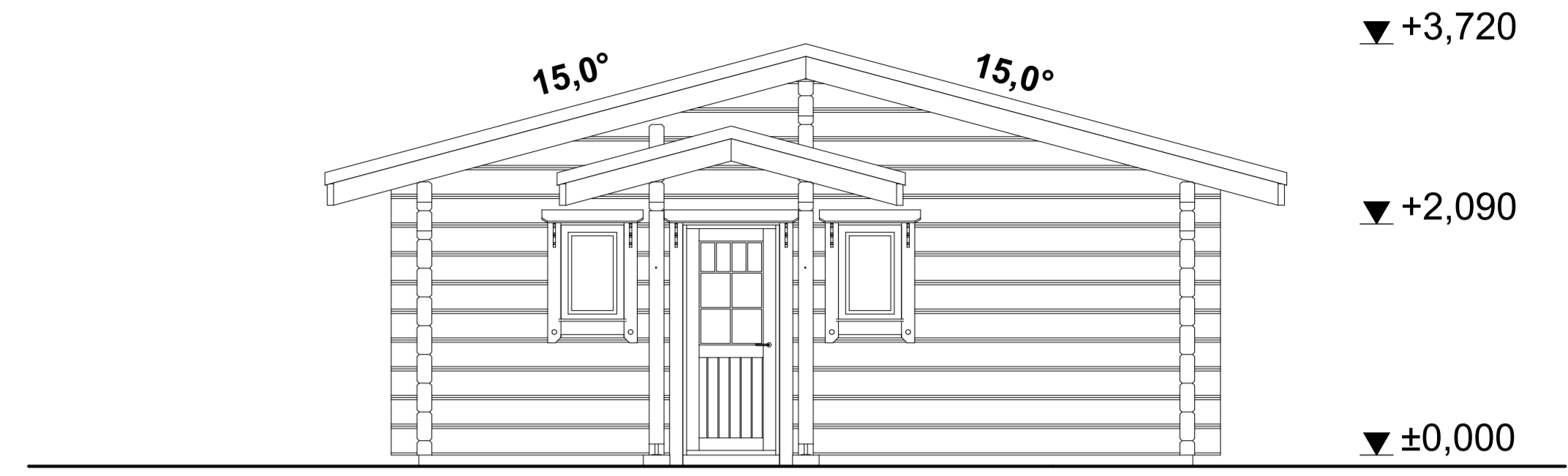
3 ELEVATION M-G julkisivu
