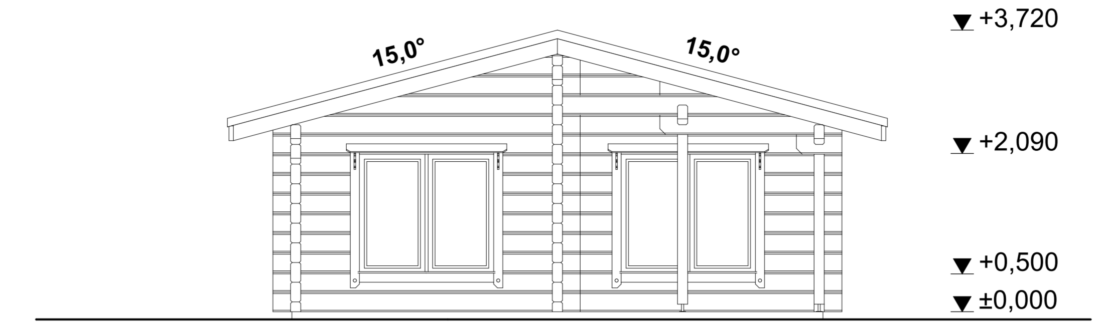
1 ELEVATION G-M julkisivu
