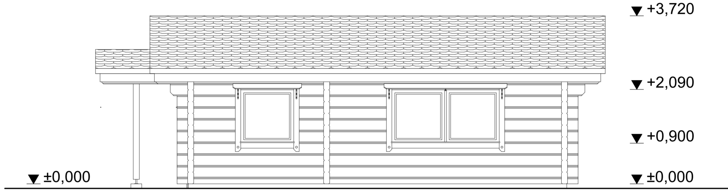
2 ELEVATION E-A julkisivu
