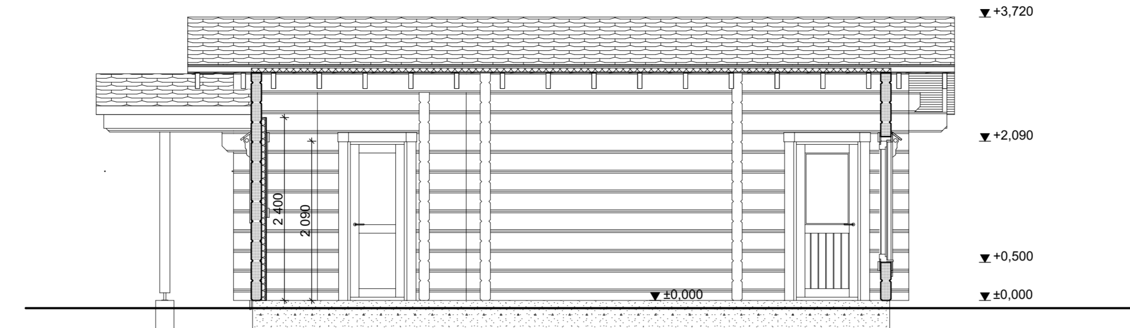
A SECTION A-A leikkaus
