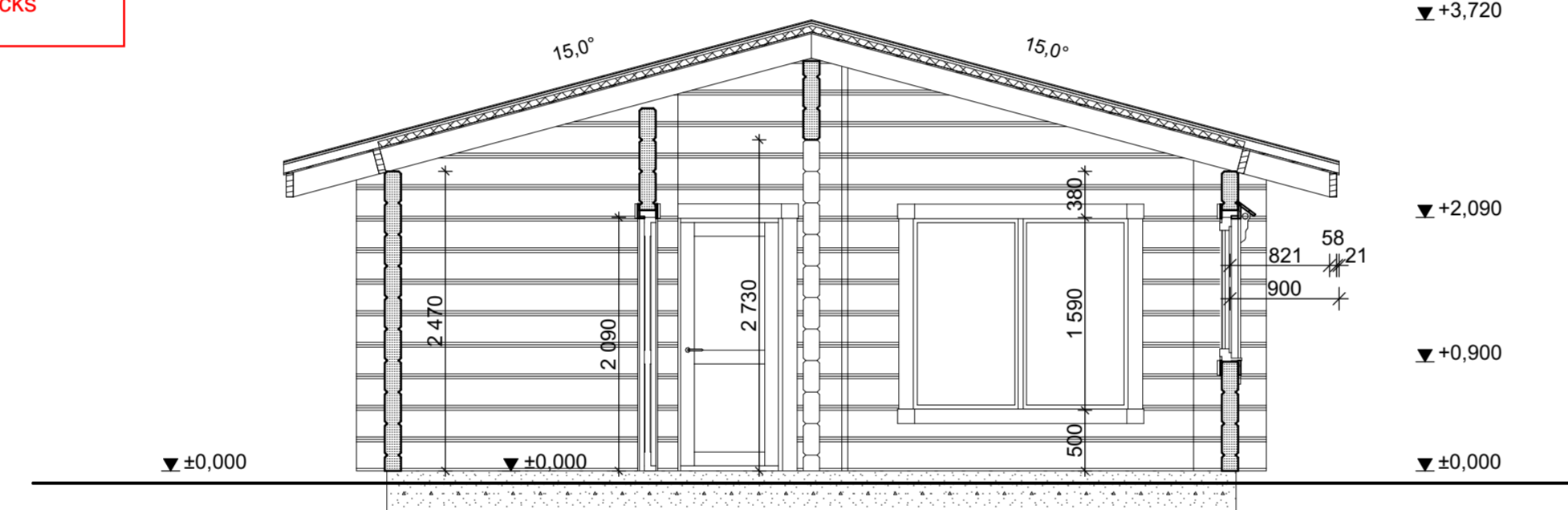
B SECTION B-B leikkaus
